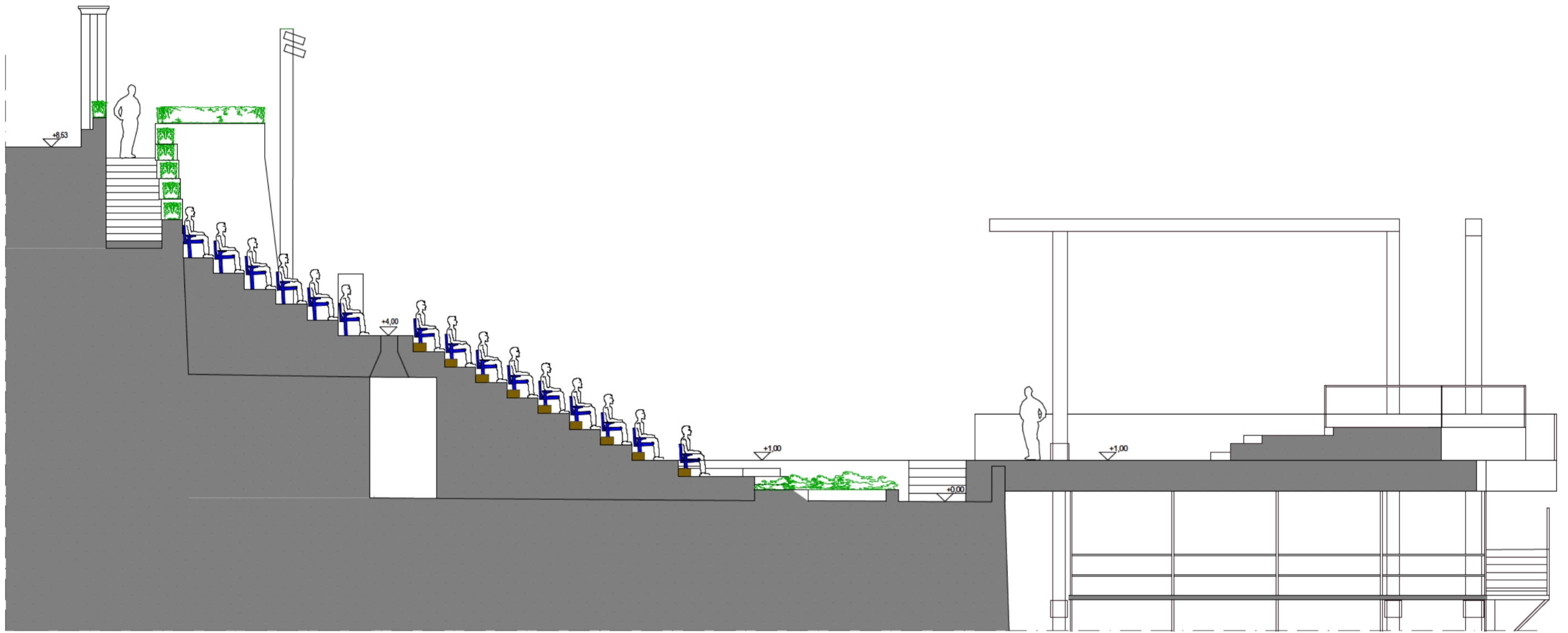
Sezione C - C
